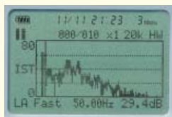
FFT分析 カード NX-22FT
