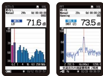
1/3オクターブ分析表示(低域)
